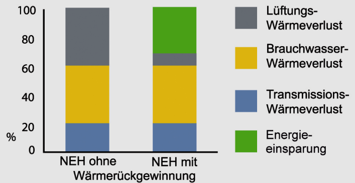
Energieeinsparung bei einem Niedrigenergiehaus (NEH).
